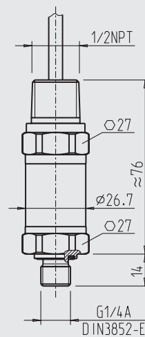
带电缆出线盒 (带1/2 NPT导线管)
